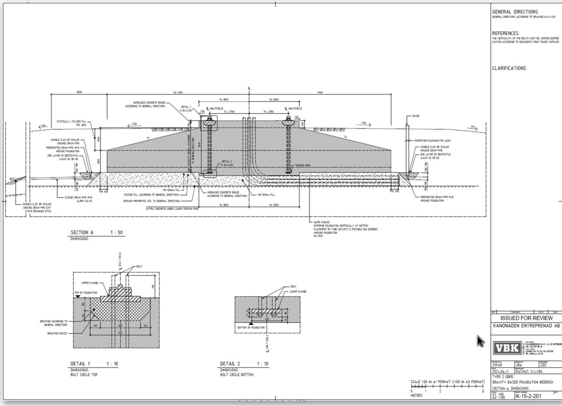
Bild: Principskiss, gravitationsfundament (Källa: Kanonaden Entreprenad AB / VBK Konsulterande Ingenjörer AB)
